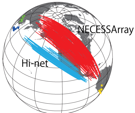
図3 南米で起きた地震を NECESSArray と日本列島で観測する場合の内核を通過する波線。北米大陸下の広範囲がサンプルされることがわかる。
