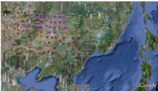
図1 NECESSArray 観測網
