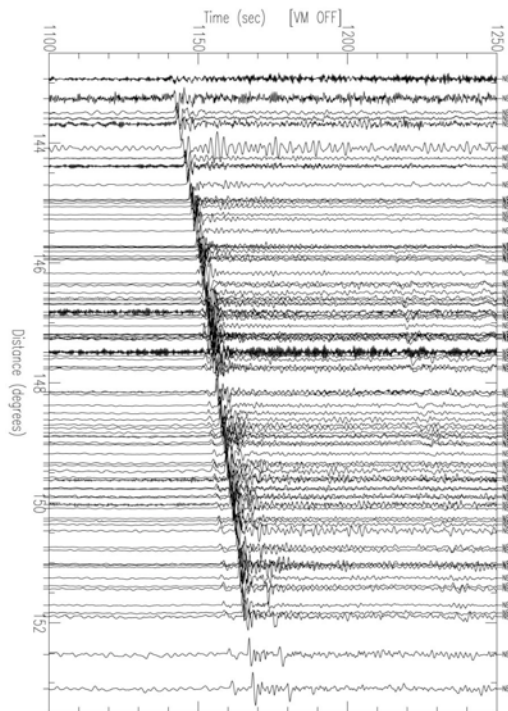
図2 NECESSArray の観測波形例（地球中心核を通る3つの波が明瞭に記録されている）
