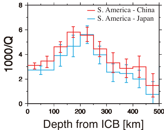
図4 NECESSArrayデータ解析等によって得られた内核の西半球の広範囲にわたって存在する可能性のある減衰構造 (Iritani 他, 2011)。東半球ではこのような特徴を持った構造は得られていないので、西半球表層から内核が成長しているというモデルとの関連が興味深い。
